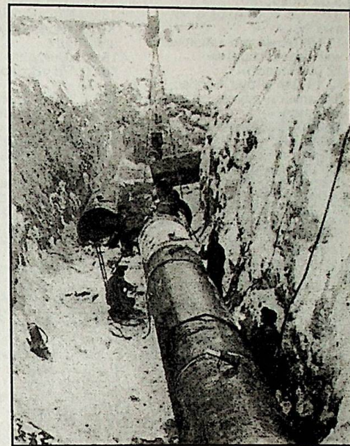
Сварочные работы на входном шлейфе КС-8. 1987 г.
